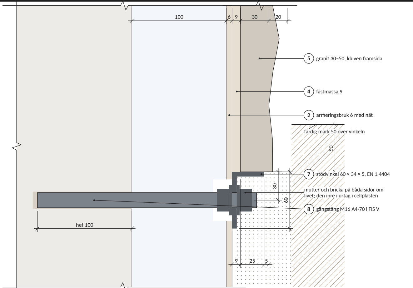
DETALJ B Stödvinkel på gängstång genom cellplasten
