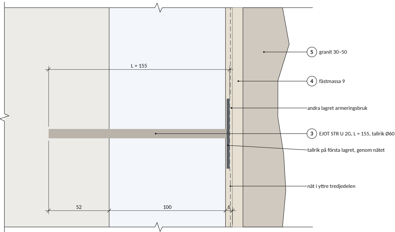
DETALJ C Armeringsbruk och isolerplugg genom nätet
